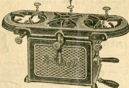
Fourneau grilloir rôtissoire à essence, à pression, sans odeur, dimensions générales 0 m 65/0 m 26/0 m 31. Dimensions de la rôtissoire 0 m 30 x 0 m 26.
