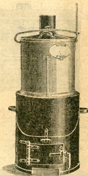
Nouveau cuiseur à vapeur en tôle noire peinte, pour l'alimentation du bétail. Contenance en litres :
