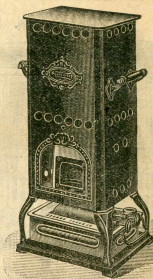
Calorifère à pétrole brûlant à flamme bleue, mèches plates. Hauteurs. . . . 0 m 56 0 m 63
