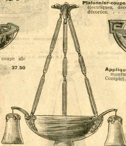
Plafonnier-coupe pâte de verre, monture bronze verni or, coupe de 0 m 40, hauteur 0 m 90, 6 lumières. Se fait en tango violet, tango bleu . . . . . 410. »
