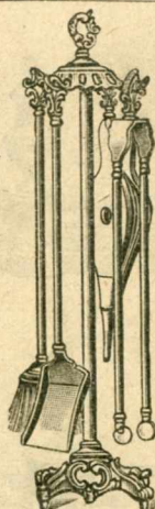
Rotonde Louis XV, cuivre vieux poli ou verni or. Hauteur 0 m 78. . . 130. »
