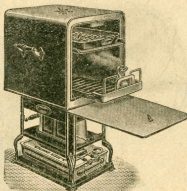
Four à double enveloppe, pour fourneaux N os 1, 2, 3. . . . . 72. »
