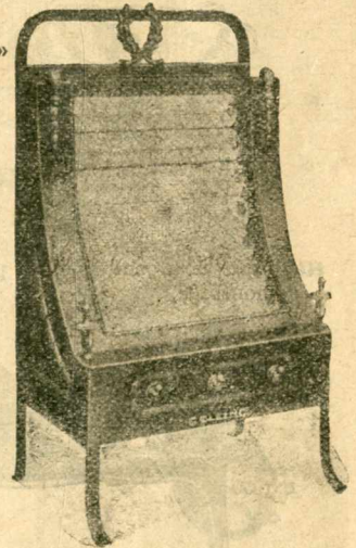
Radiateur électrique, modèle riche, en cuivre poli, réglage par interrupteur, 300, 600, 900 watts, 110 volts.
