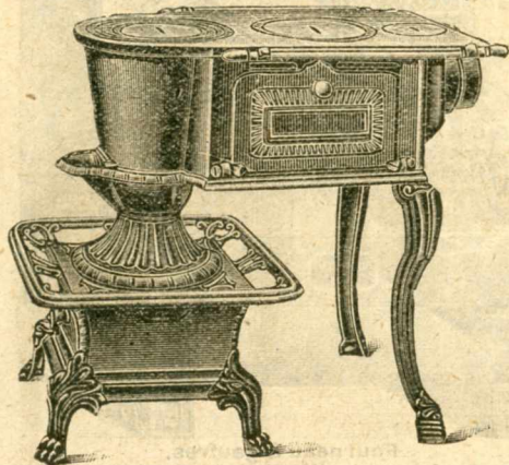
Poêle flamand "Godin", à socle, avec four, tuyau dessus ou derrière, avec galeries au socle et sur les côtés. Longueurs du dessus. 0m69 0m81 0m87 Prix . . . . . 211. » 253. » 288. »
